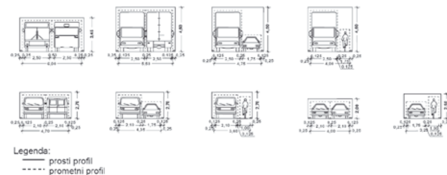
Slika 5: Dimenzije prometnih profilov za tipične sestave tipičnih vozil pri zelo majhni vozni hitrosti (40 km/h)
